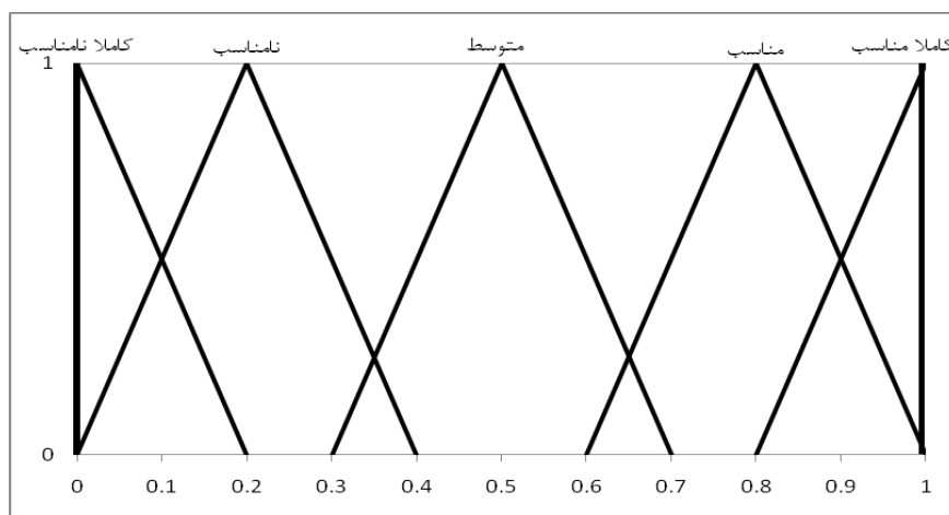
شکل ۲. طیف ۵ مقیاسی فازی در بازه {۰-۱} (کاهرامان ۲۰۰۷)
