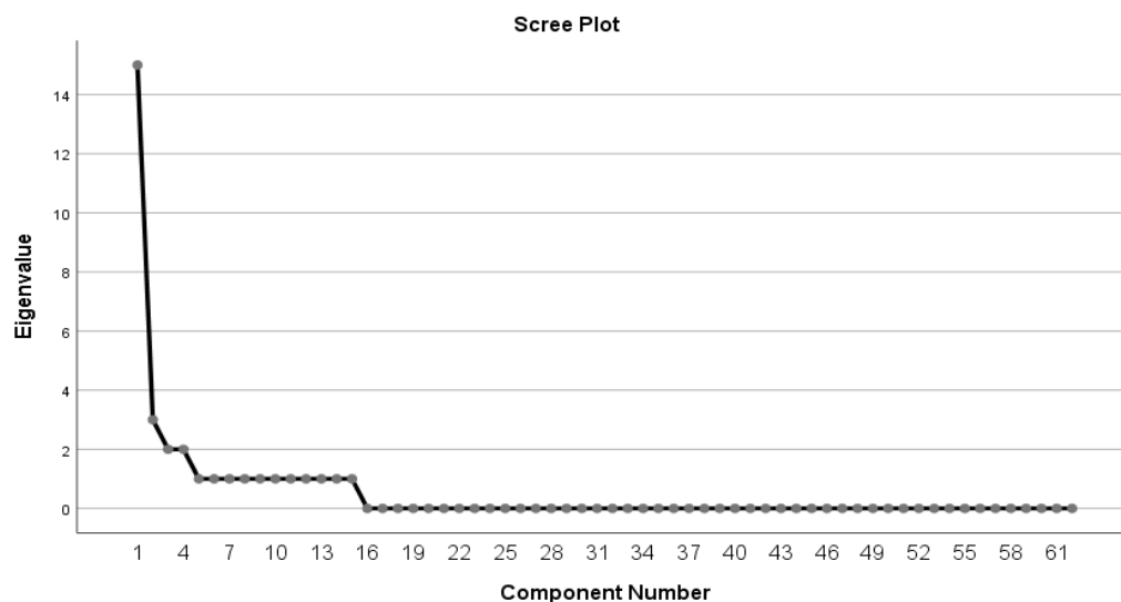
شکل ۱- نمودار اسکری کنترل برای مؤلفه‌های استخراجی پرسش‌نامه
