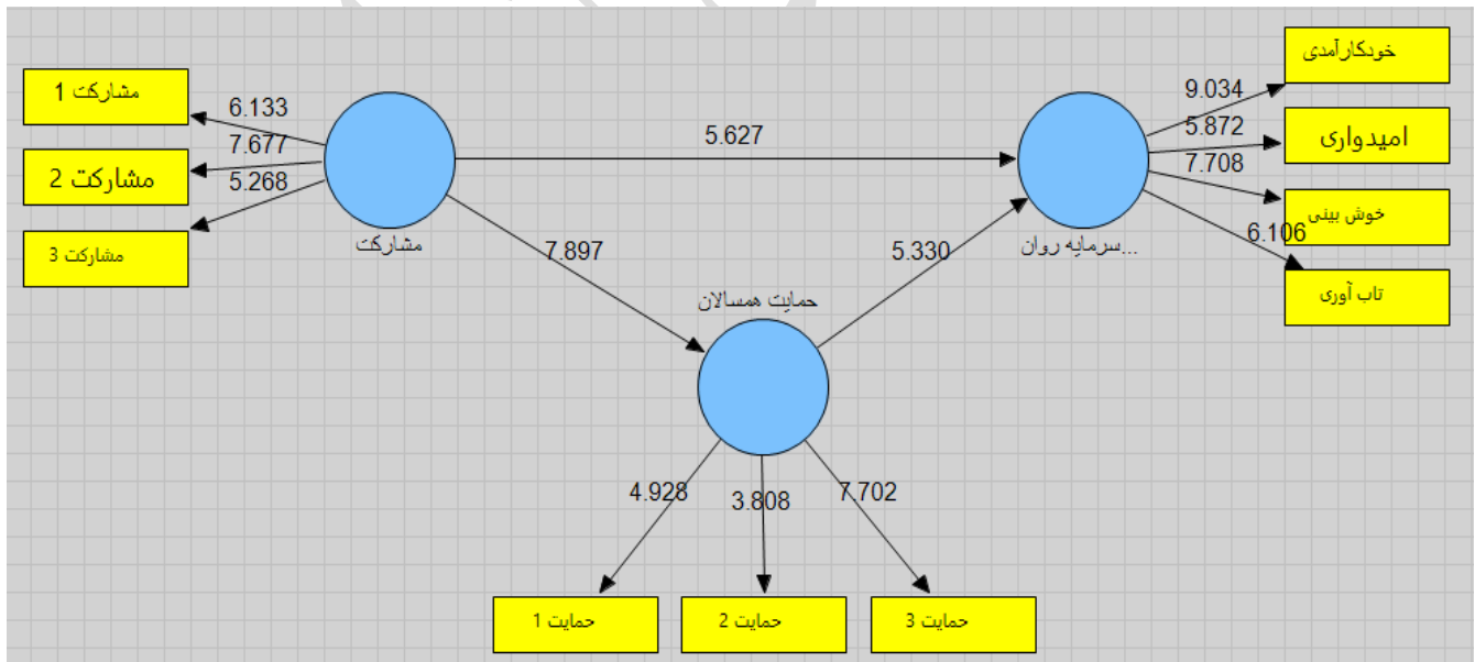
شکل ۲- مدل پژوهش در حالت میزان تی
