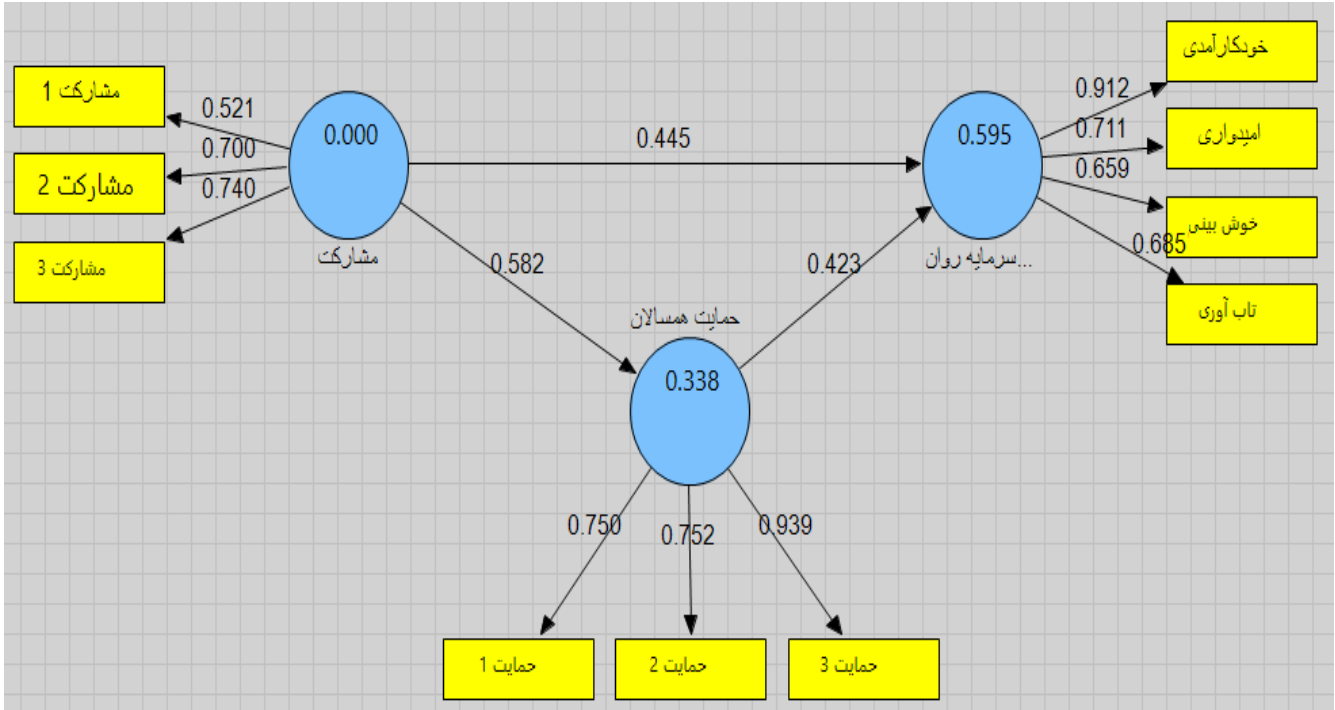
شکل ۱- مدل پژوهش در حالت ضرایب مسیر
